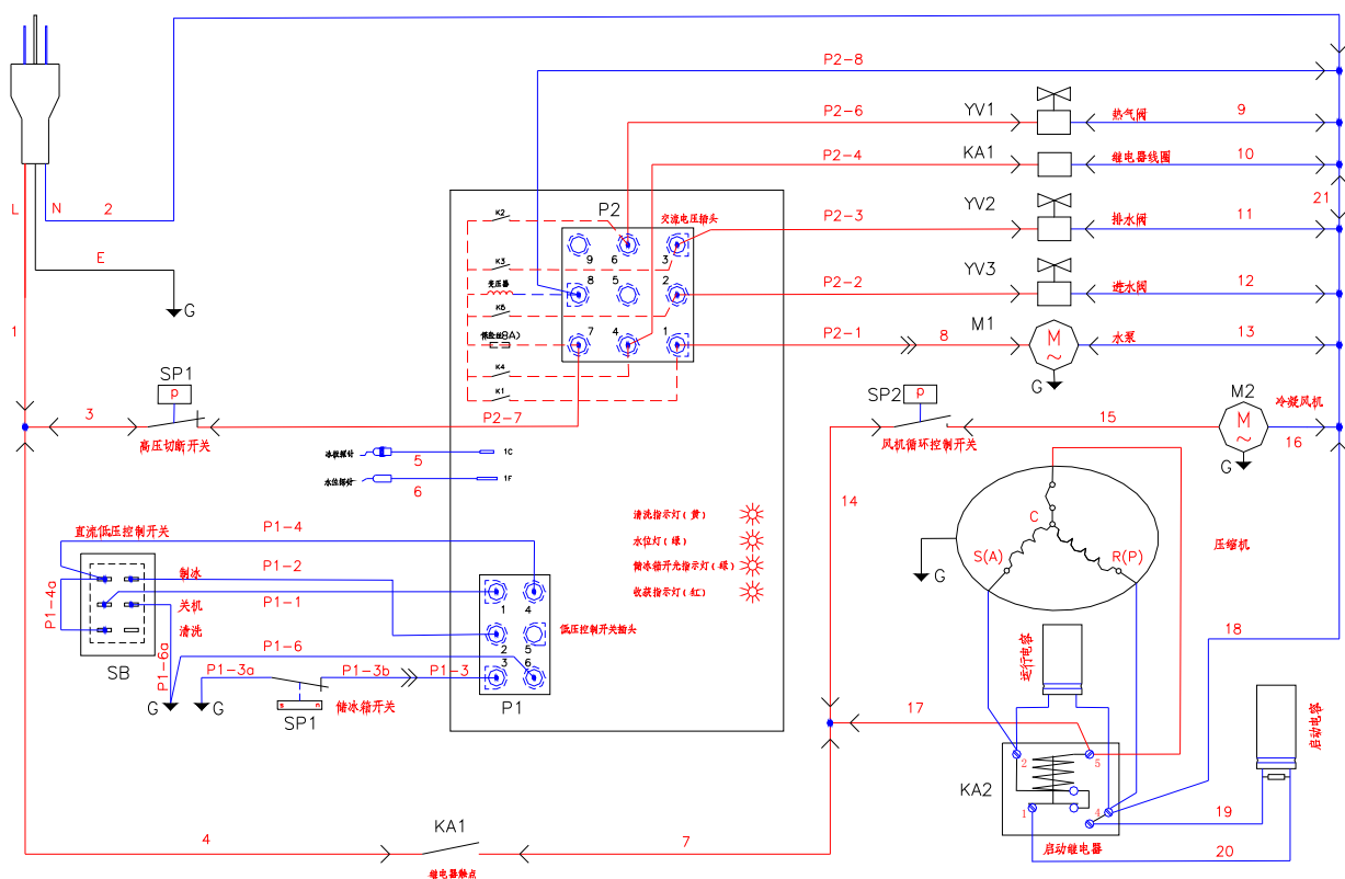
CM-215 接線圖
