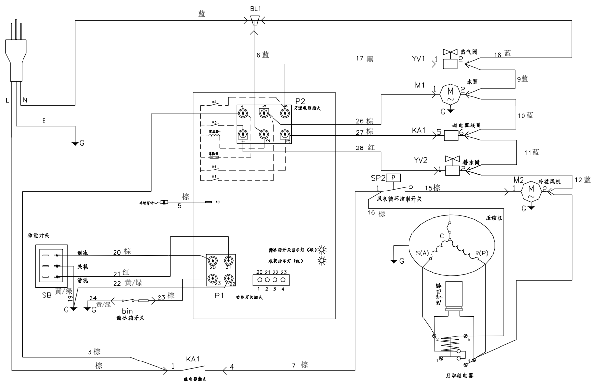
CM-105 接線圖
