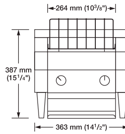
正視圖
