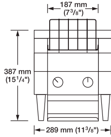
正視圖
