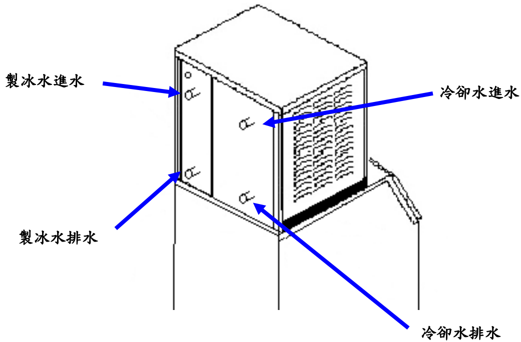
進排水管路配置
